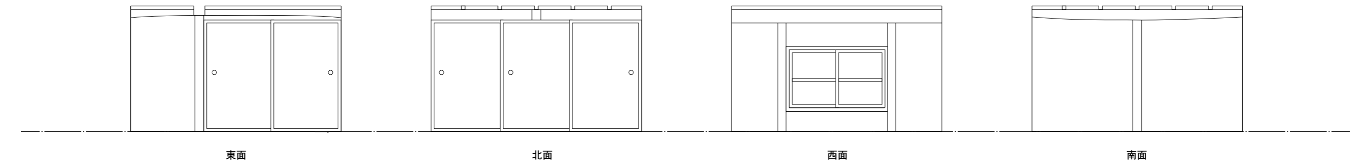
2階監視部屋展開図
