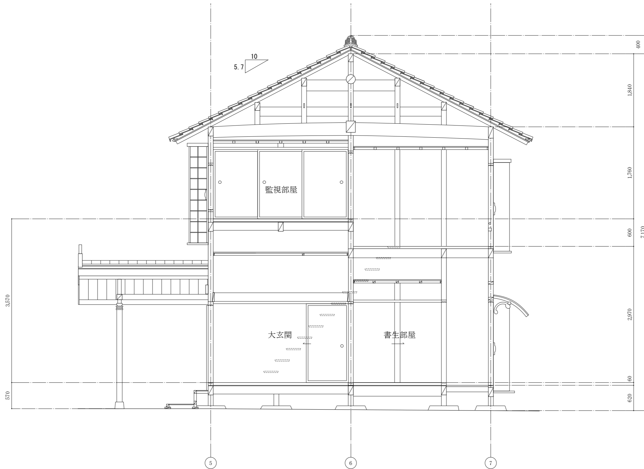
A-A' 断面図
