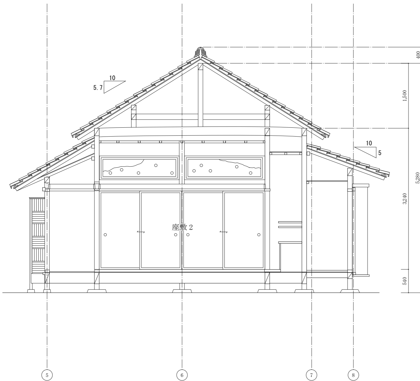
B-B' 断面図
