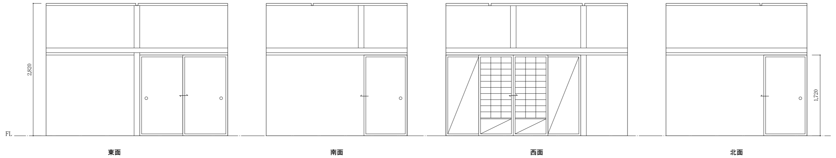
大玄関展開図
