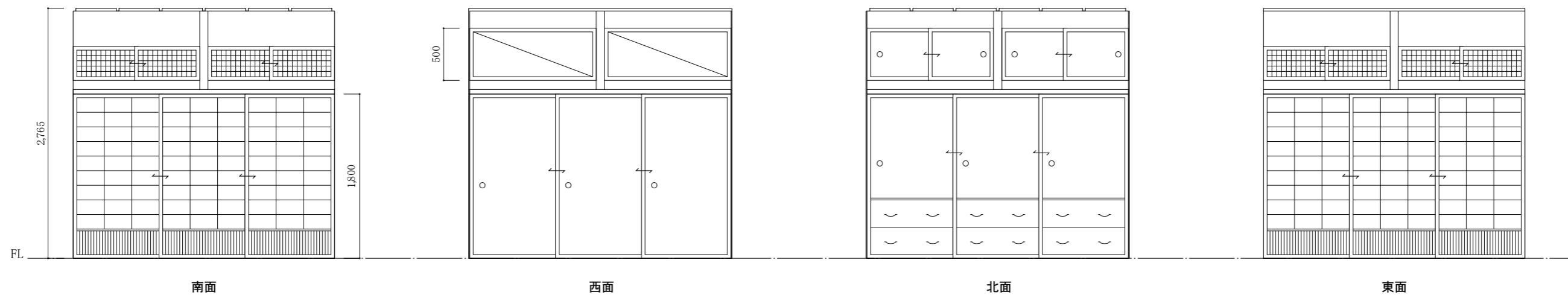
次の間展開図
