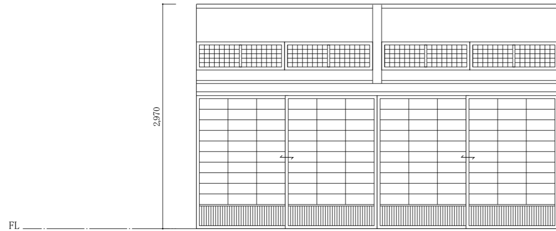
西面
