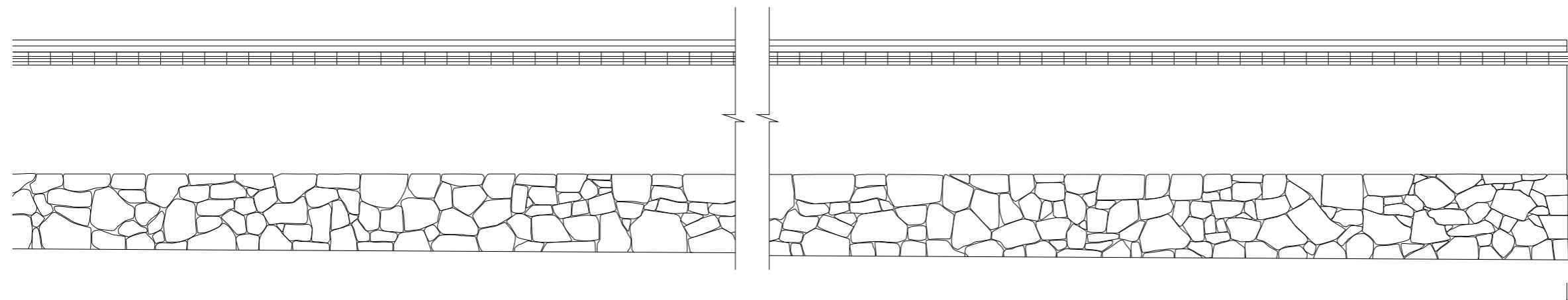
築地塀南面立面図
