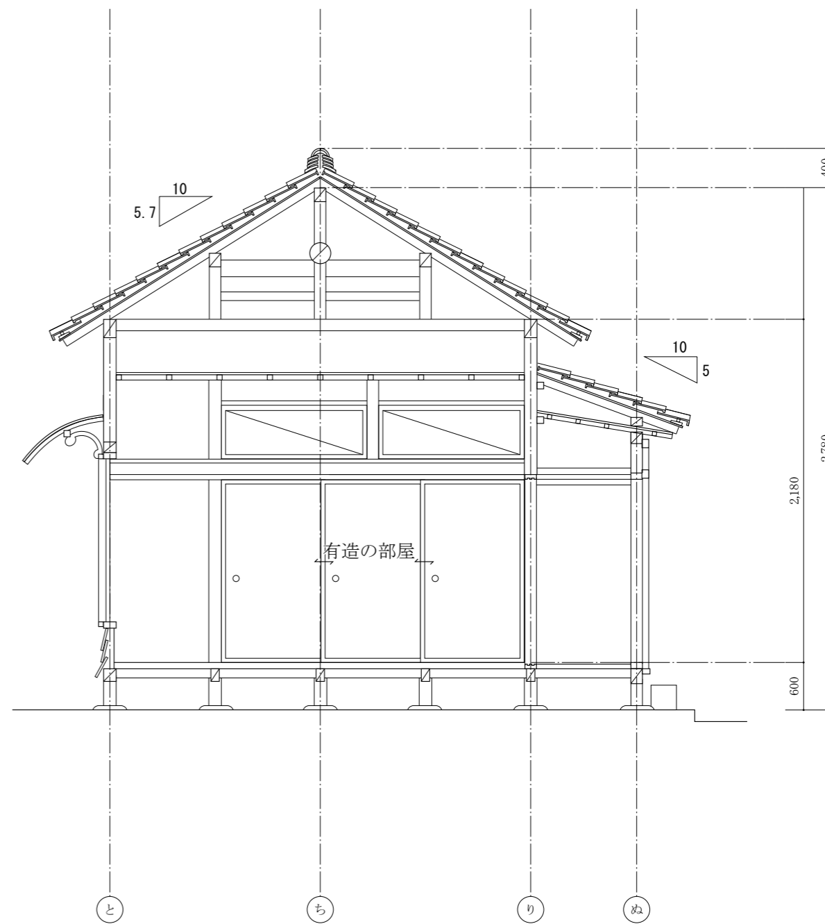
C-C' 断面図
