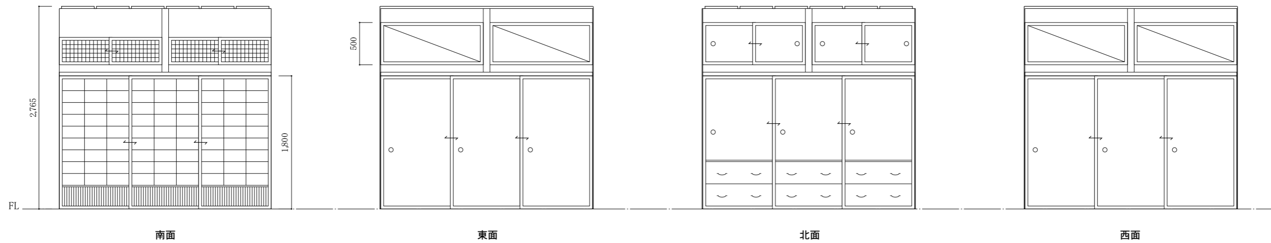
有造の部屋展開図
