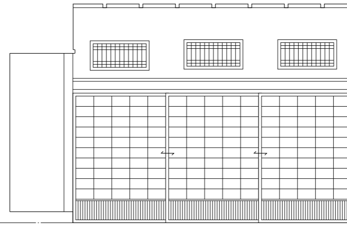
南面
