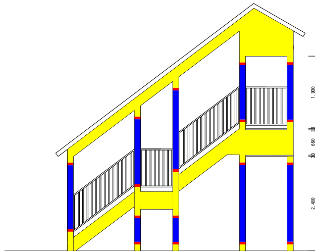
立面図②
