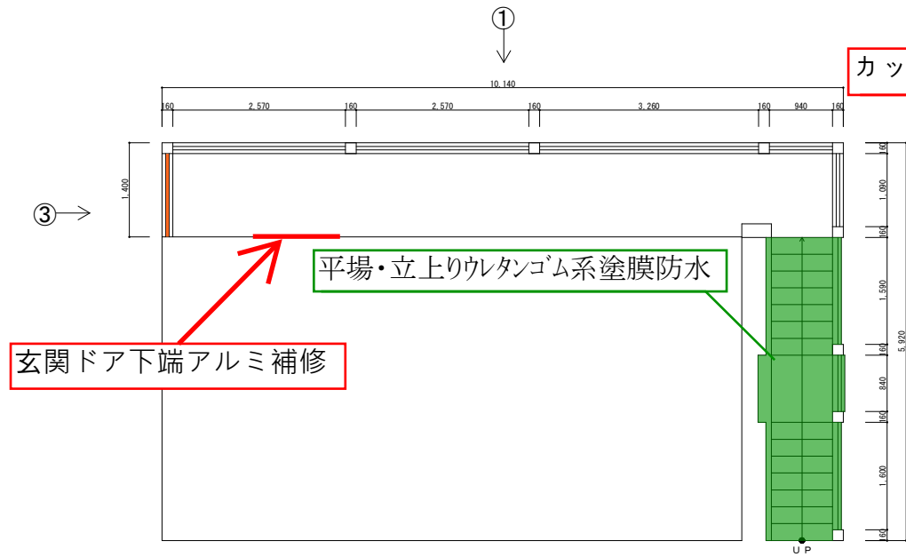
平面図
