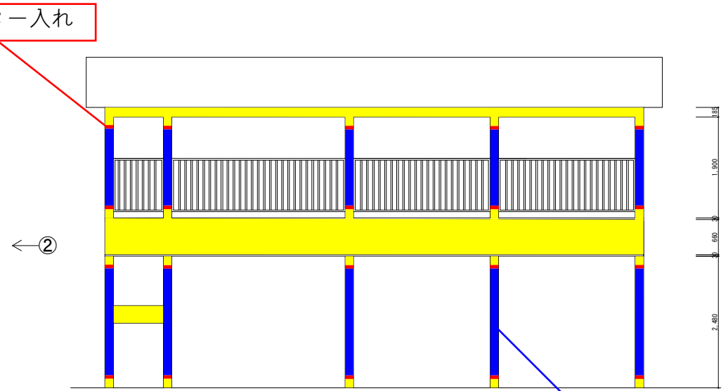
立面図①
