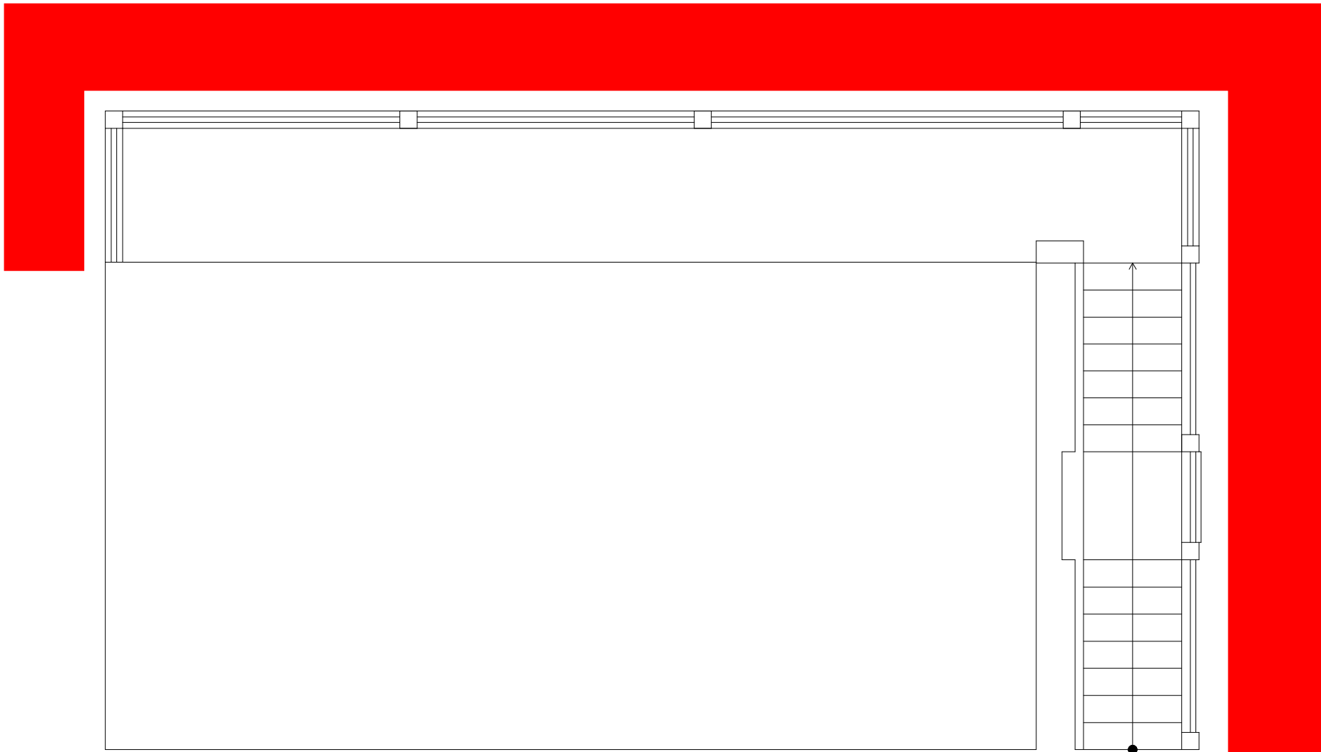
足場計画図
