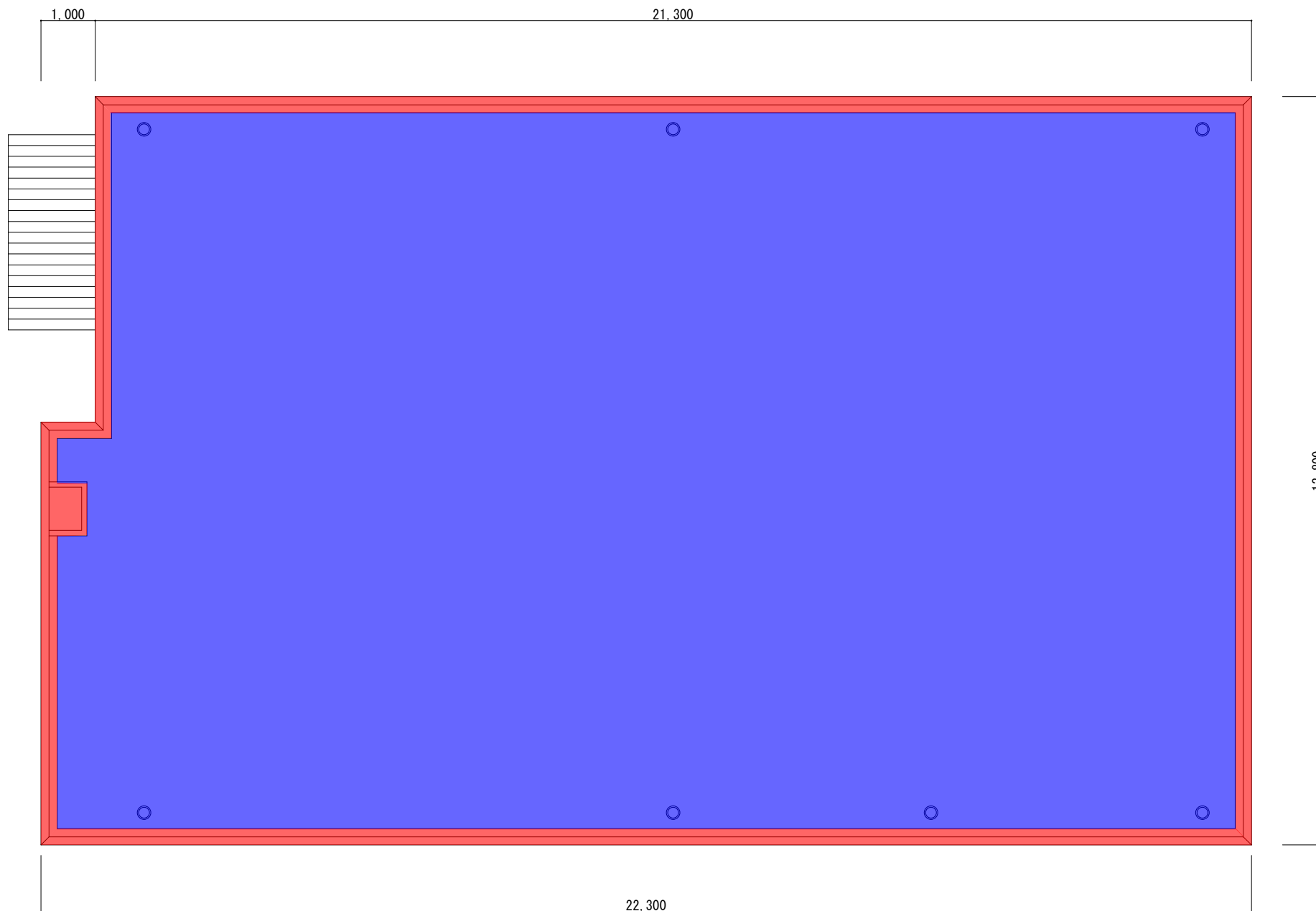
平面図 1/100
