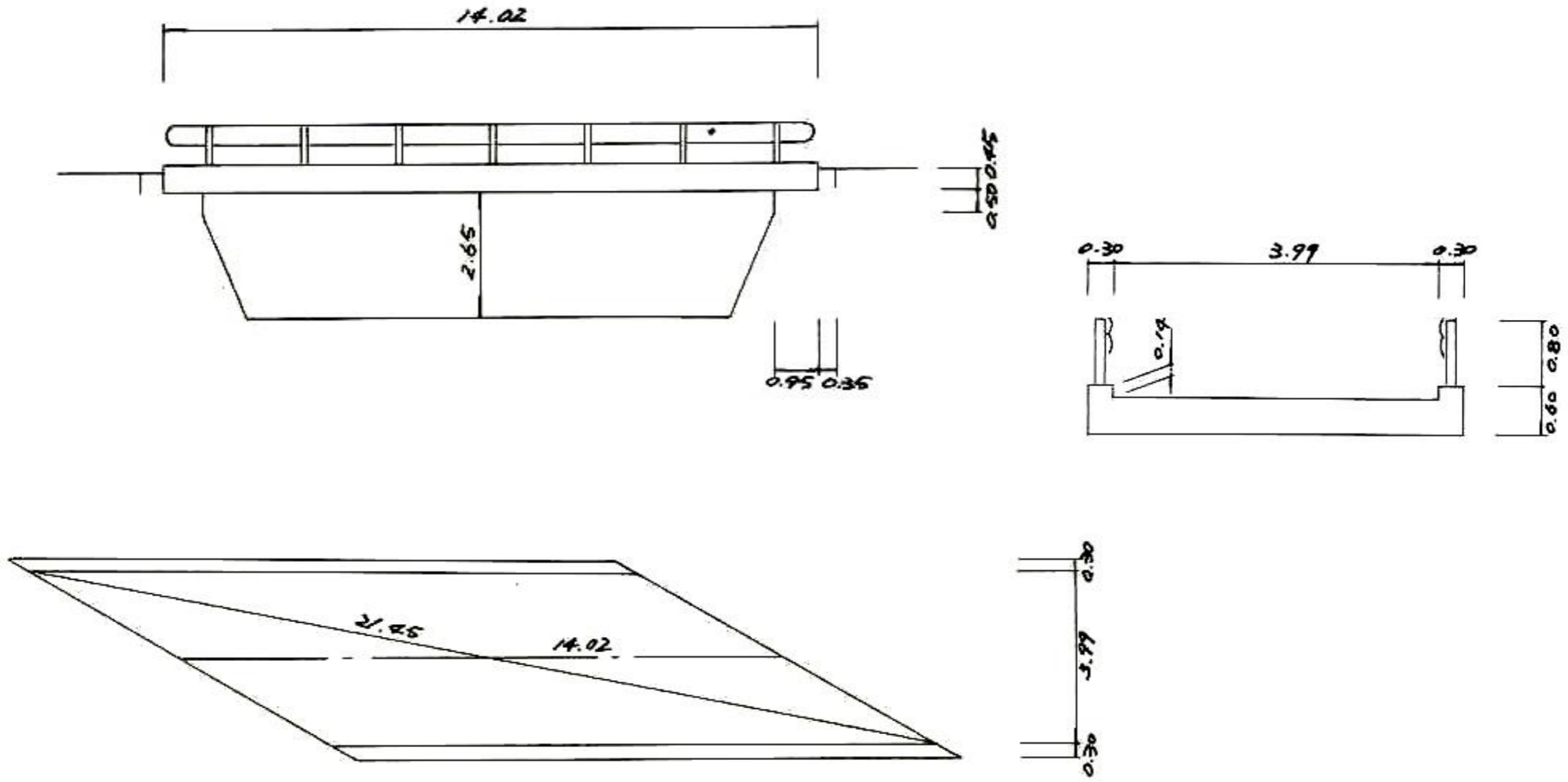
橋梁一般図
