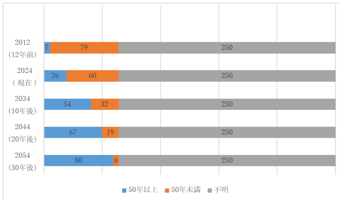
高齢化橋梁の推移
