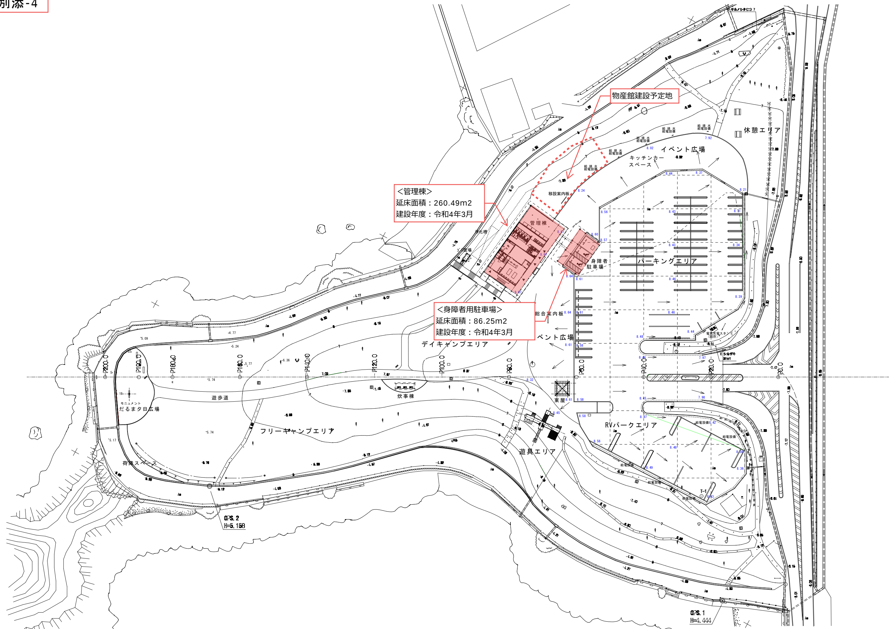
既存建物配置図・平面図
