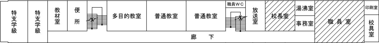
2階平面図
